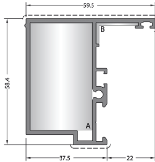
CODE / KOD 58C-502-18 THEORETICAL WEIGHT kg/m TEORİK AĞIRLIK kg/m 1.136
