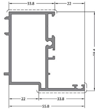
CODE / KOD 58C-404-00 THEORETICAL WEIGHT kg/m TEORİK AĞIRLIK kg/m 1.139
