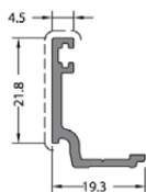
CODE / KOD 07-111-00 THEORETICAL WEIGHT kg/m TEORİK AĞIRLIK kg/m 0.234
