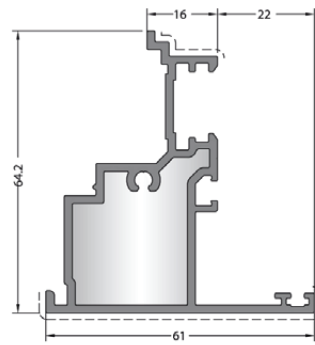
CODE / KOD 58C-501-18 THEORETICAL WEIGHT kg/m TEORİK AĞIRLIK kg/m 1.164
